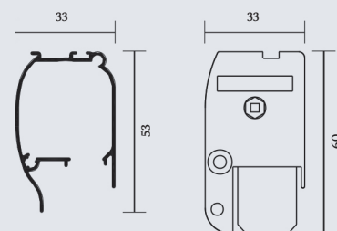
Mesures caisson avec embout SR33 (À visser) Kassettengröße mit Endkappe SR33 (Zum Schrauben)
