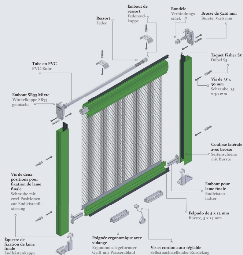
Vue éclatée Mosquitera SR33 fenêtre Explosionsgrafik Rollo SR33 Fenster
